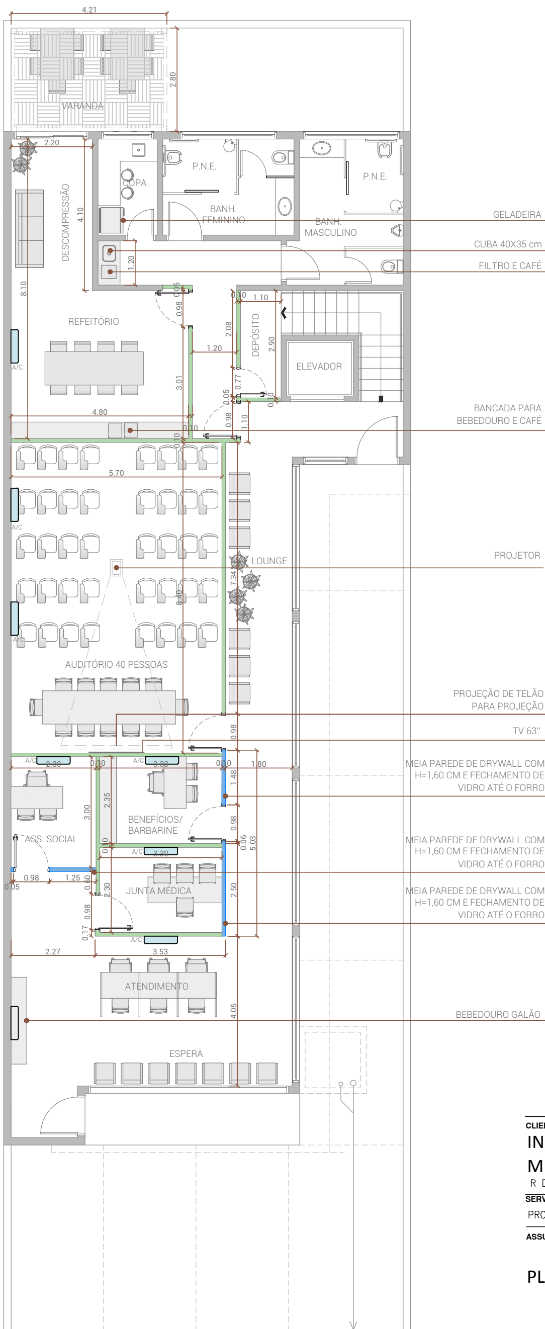
PLANTA TÉRREO ESC. 1:100
